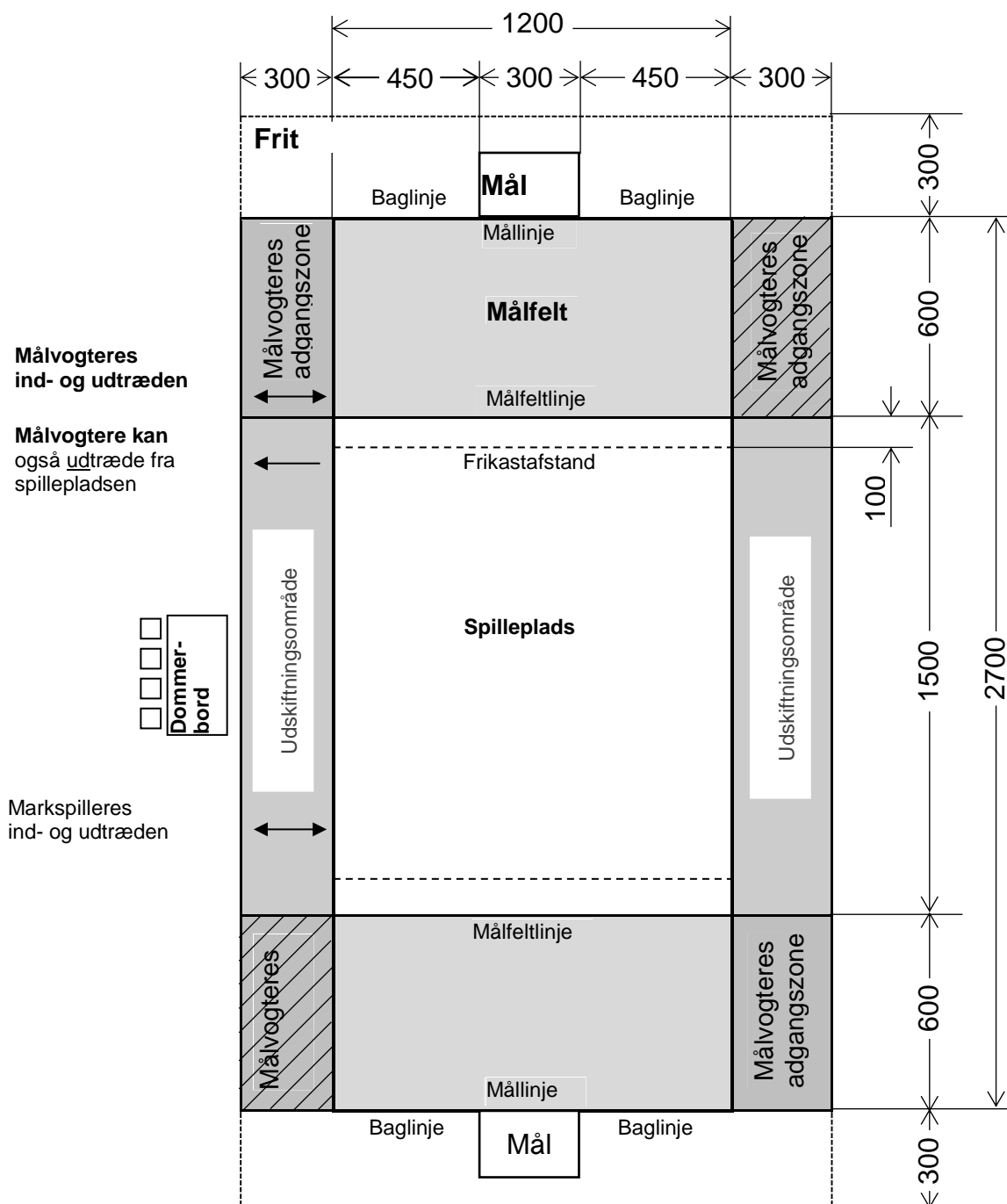
Figur 1: Beach Handball banen (Alle målangivelser er i cm)
